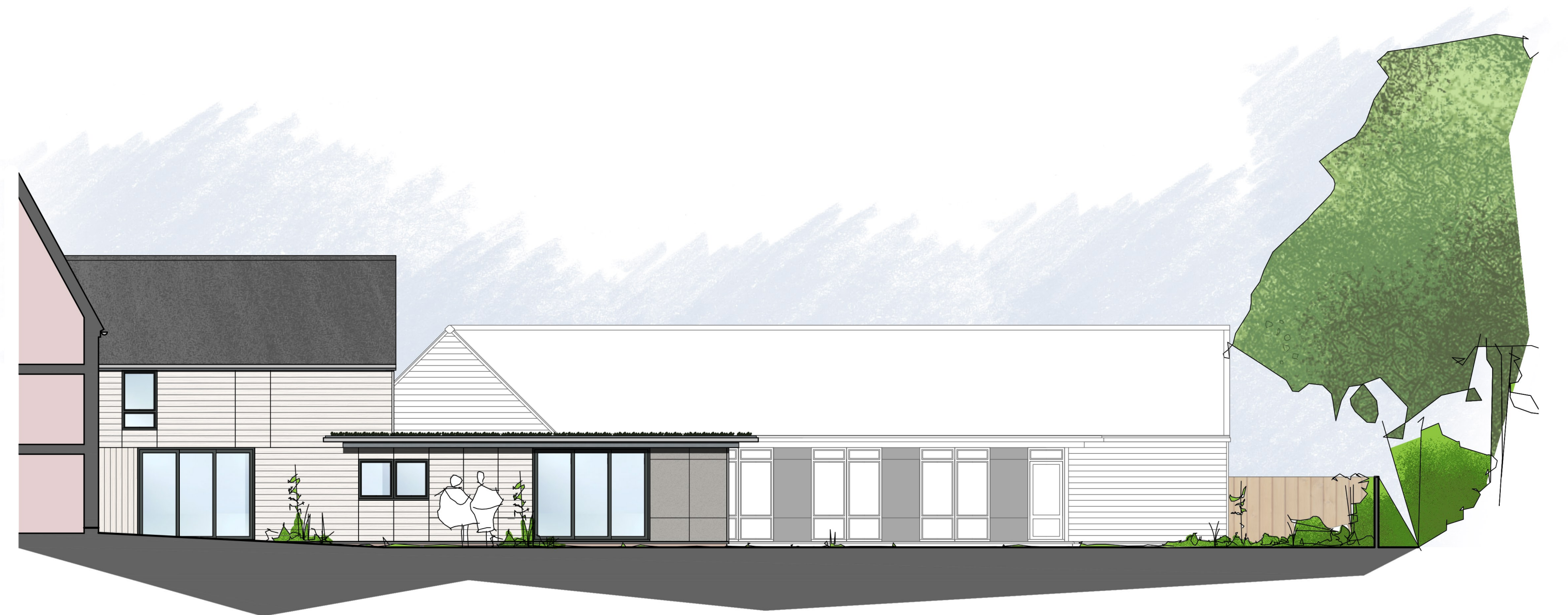
Elevation G-G
